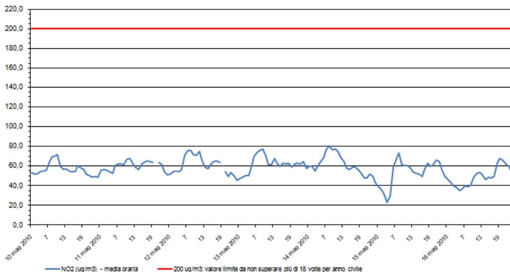
Biossido di azoto - NO 2 Stazione di rilevamento di via B. Cairoli, periodo: 10 mag 2010 - 16 mag 2010
