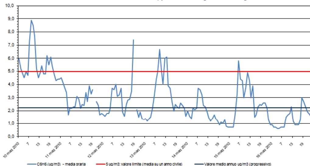
Benzene - C 6 H 6 Stazione di rilevamento di via B. Cairoli, periodo: 10 mag 2010 - 16 mag 2010
