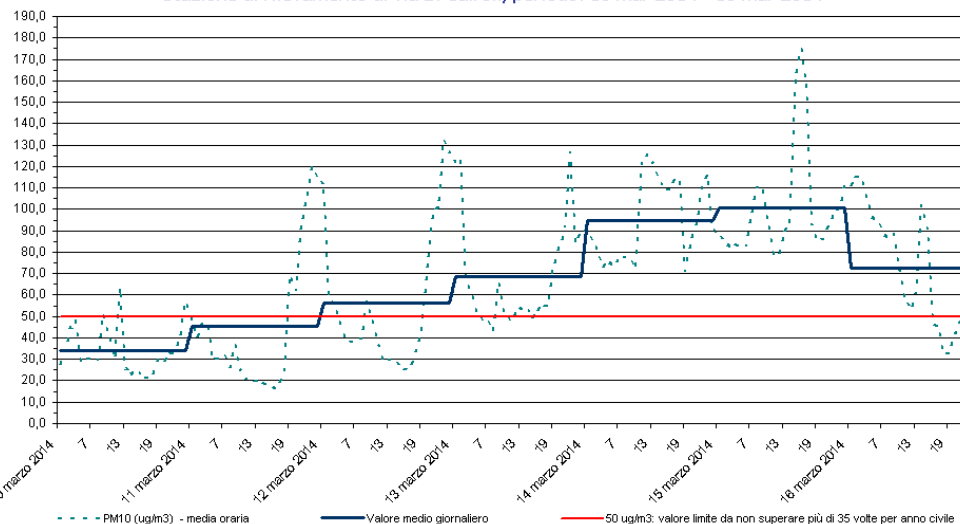
PM10 Stazione di rilevamento di via B. Cairoli, periodo: 10 mar 2014 - 16 mar 2014
