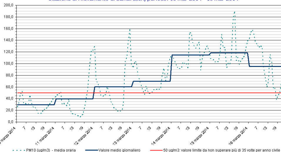
PM10 Stazione di rilevamento di Sambruson, periodo: 10 mar 2014 - 16 mar 2014
