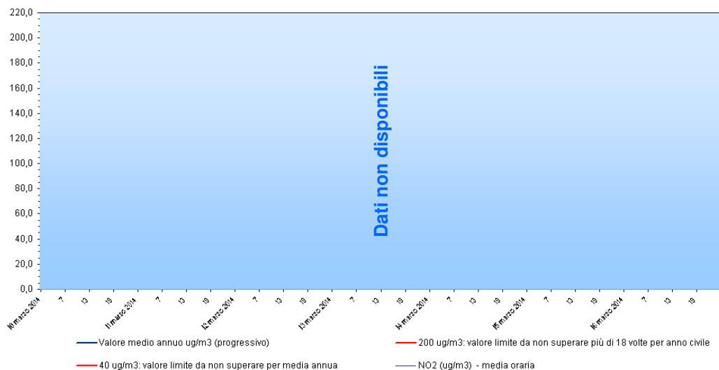
Biossido di azoto - NO 2 Stazione di rilevamento di Sambruson, periodo: 10 mar 2014 - 16 mar 2014
