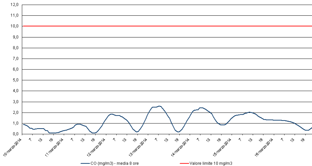
Monossido di Carbonio - CO Stazione di rilevamento di Sambruson, periodo: 10 mar 2014 - 16 mar 2014
