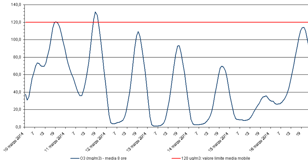
Ozono - O 3 Stazione di rilevamento di Sambruson, periodo: 10 mar 2014 - 16 mar 2014
