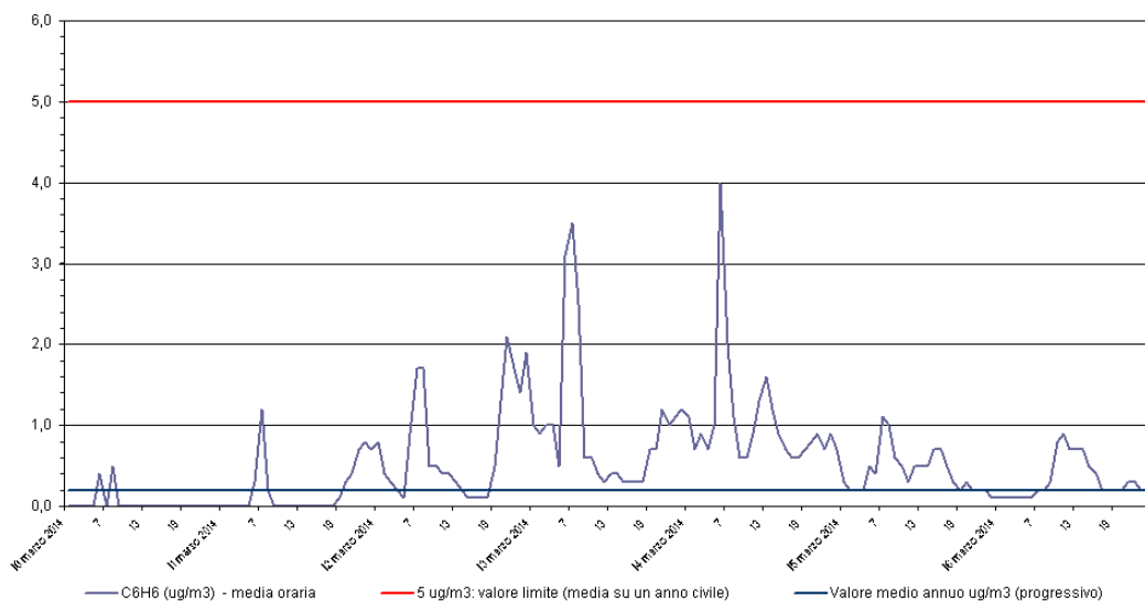
Benzene - C 6 H 6 Stazione di rilevamento di Sambruson, periodo: 10 mar 2014 - 16 mar 2014
