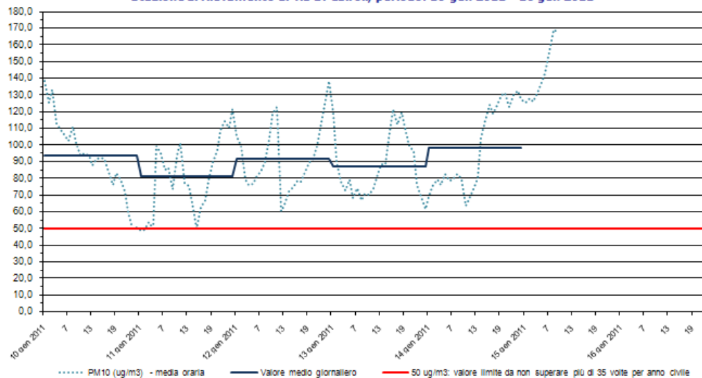
PM10 Stazione di rilevamento di via B. Cairoli, periodo: 10 gen 2011 - 16 gen 2011
