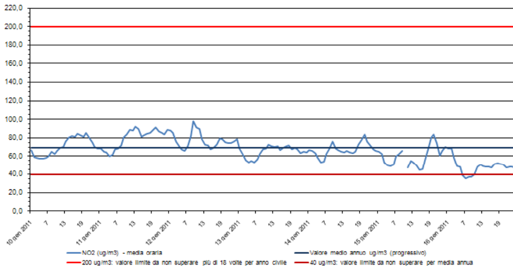
Biossido di azoto - NO 2 Stazione di rilevamento di via B. Cairoli, periodo: 10 gen 2011 - 16 gen 2011
