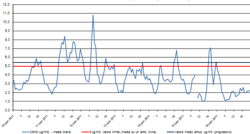
Benzene - C 6 H 6 Stazione di rilevamento di via B. Cairoli, periodo: 10 gen 2011 - 16 gen 2011
