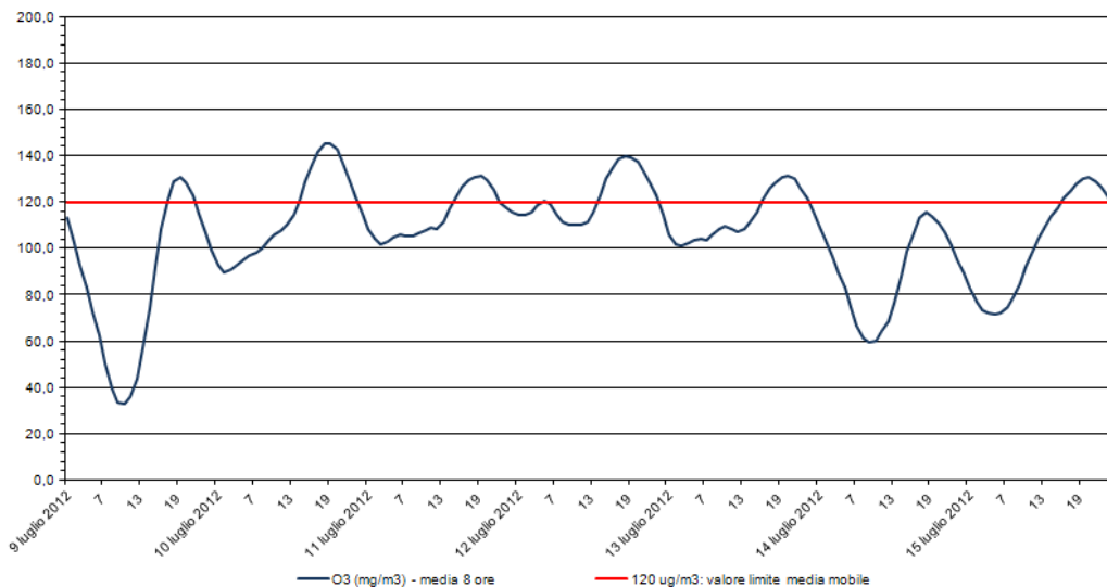
Ozono - O3 Stazione di rilevamento di via B. Cairoli, periodo: 09 lug 2012- 15 lug 2012
