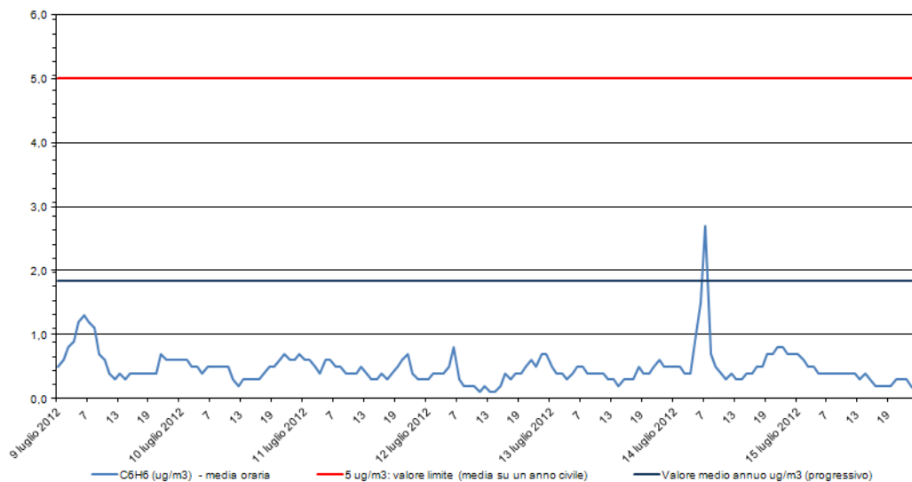
Benzene - C 6 H 6 Stazione di rilevamento di via B. Cairoli, periodo: 09 lug 2012- 15 lug 2012
