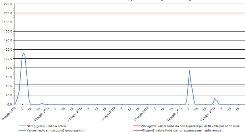
Biossido di azoto - NO 2 Stazione di rilevamento di via B. Cairoli, periodo: 09 lug 2012- 15 lug 2012
