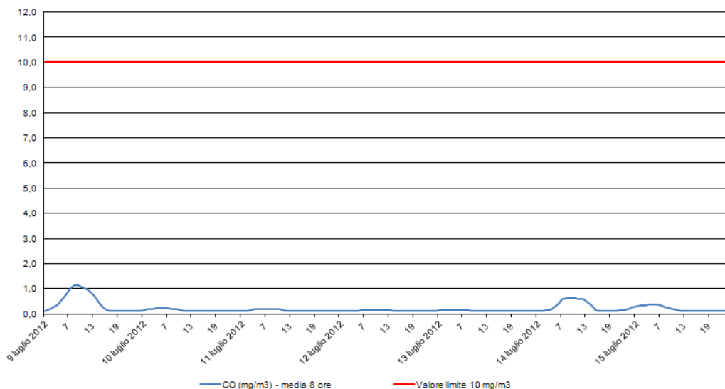
Monossido di Carbonio - CO Stazione di rilevamento di via B. Cairoli, periodo: 09 lug 2012- 15 lug 2012
