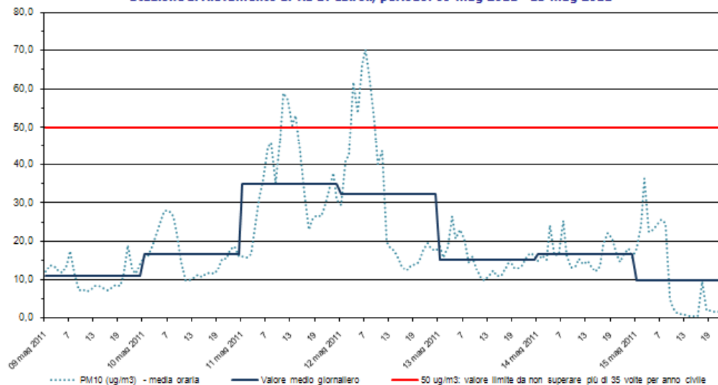
PM10 Stazione di rilevamento di via B. Cairoli, periodo: 09 mag 2011 - 15 mag 2011
