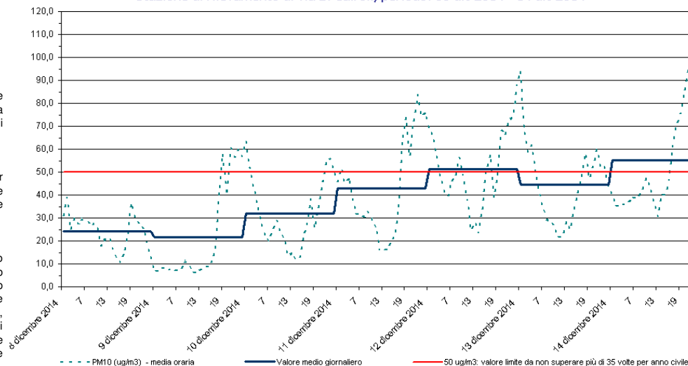
PM10 Stazione di rilevamento di via B. Cairoli, periodo: 08 dic 2014 - 14 dic 2014
