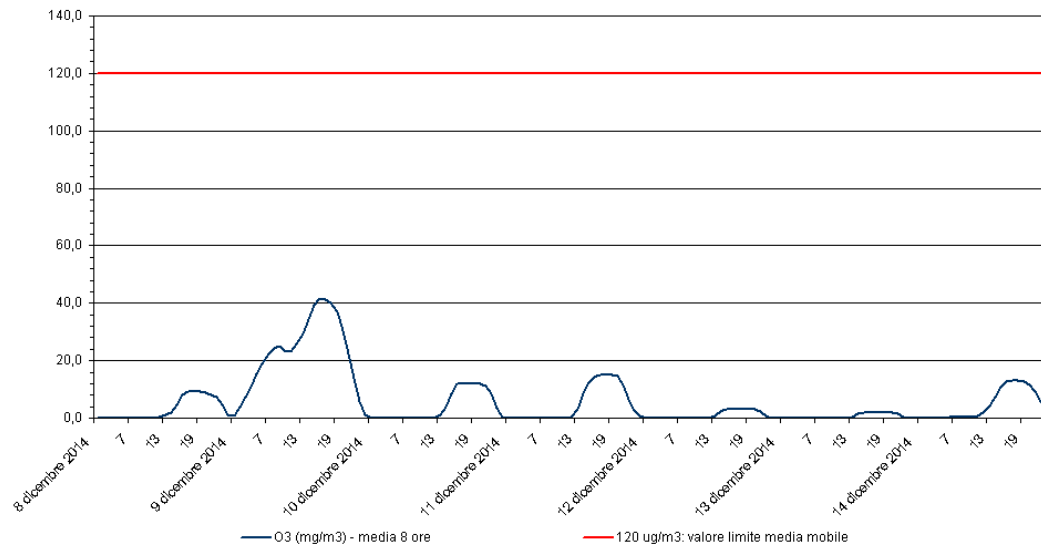
Ozono - O 3 Stazione di rilevamento di Sambruson, periodo: 08 dic 2014 - 14 dic 2014
