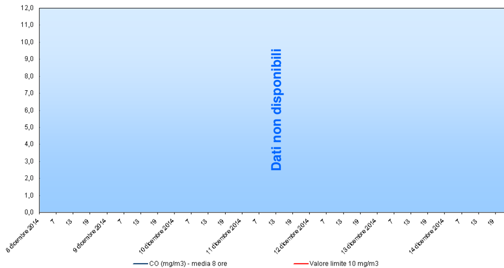
Monossido di Carbonio - CO Stazione di rilevamento di Sambruson, periodo: 08 dic 2014 - 14 dic 2014
