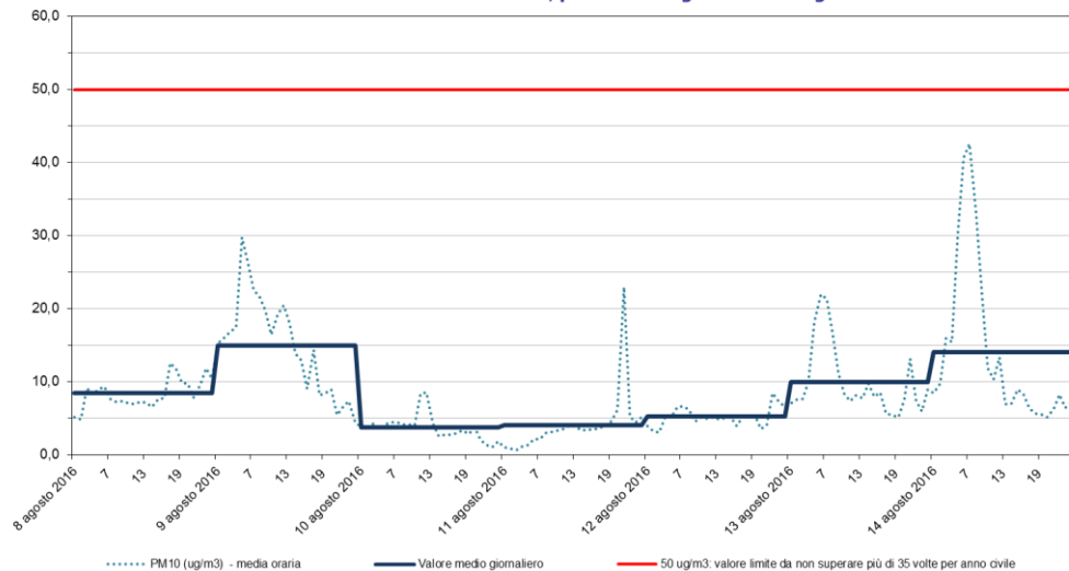
PM10 Stazione di rilevamento di via B. Cairoli, periodo: 08 ago 2016 - 14 ago 2016
