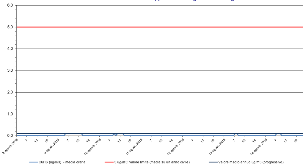
Benzene - C 6 H 6 Stazione di rilevamento di Sambruson, periodo: 08 ago 2016 - 14 ago 2016
