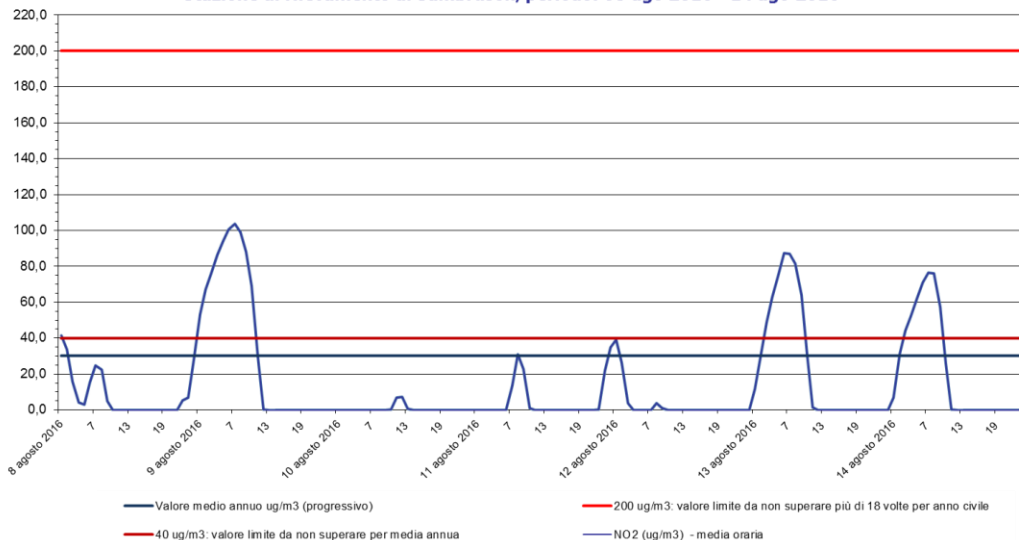
Biossido di azoto - NO 2 Stazione di rilevamento di Sambruson, periodo: 08 ago 2016 - 14 ago 2016
