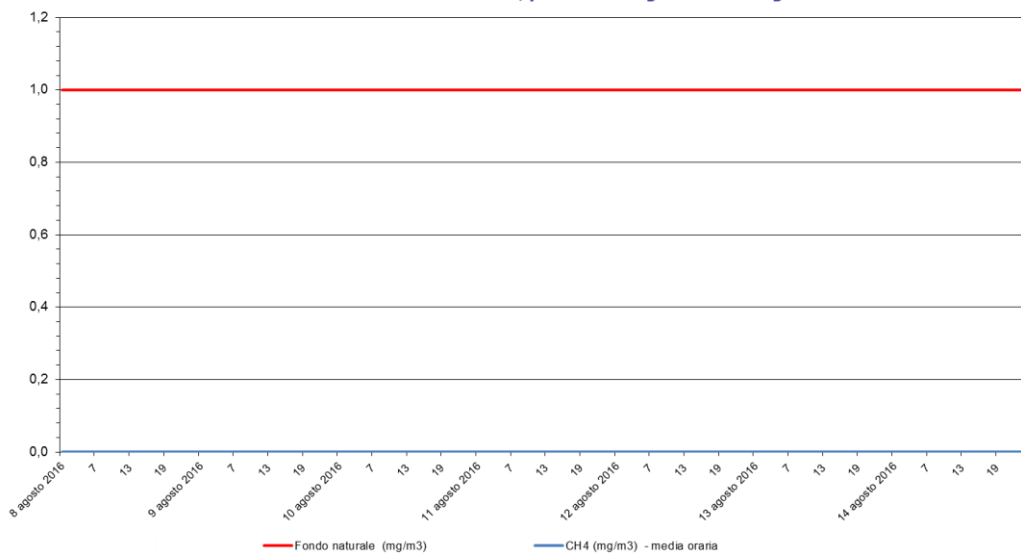
Metano - CH 4 Stazione di rilevamento di Sambruson, periodo: 08 ago 2016 - 14 ago 2016
