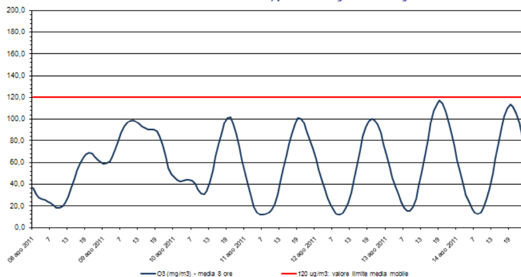
Ozono - O3 Stazione di rilevamento di via B. Cairoli, periodo: 08 ago 2011 - 14 ago 2011
