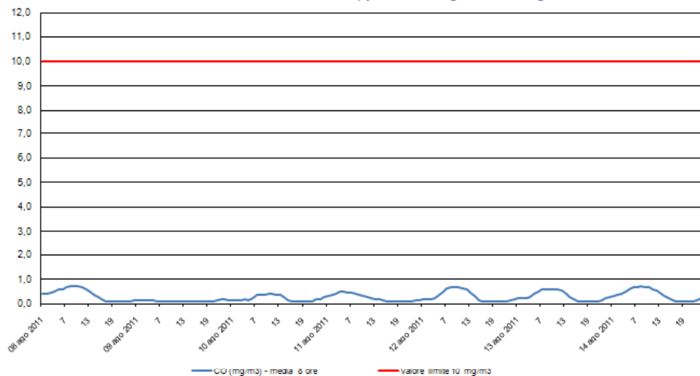
Monossido di Carbonio - CO Stazione di rilevamento di via B. Cairoli, periodo: 08 ago 2011 - 14 ago 2011
