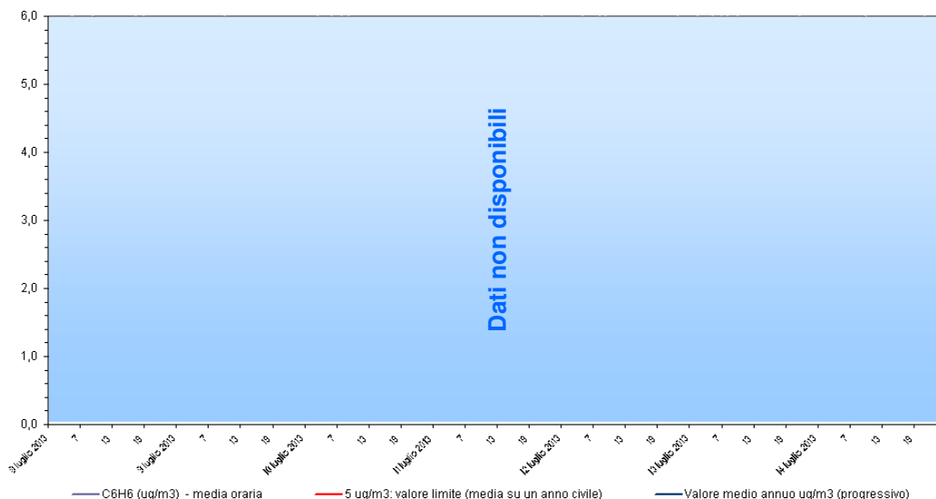
Benzene - C 6 H 6 Stazione di rilevamento di Sambruson, periodo: 08 lug 2013 - 14 lug 2013
