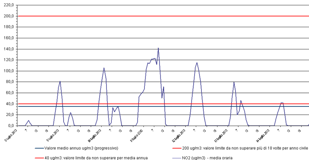
Biossido di azoto - NO 2 Stazione di rilevamento di Sambruson, periodo: 08 lug 2013 - 14 lug 2013
