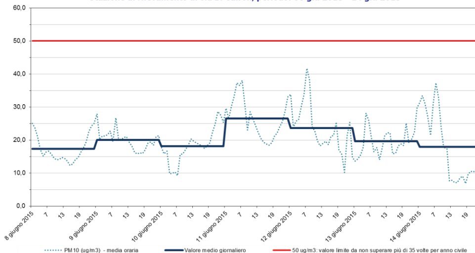
PM10 Stazione di rilevamento di via B. Cairoli, periodo: 08 giu 2015 - 14 giu 2015
