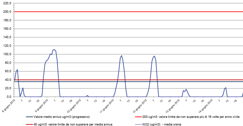
Biossido di azoto - NO 2 Stazione di rilevamento di Sambruson, periodo: 08 giu 2015 - 14 giu 2015
