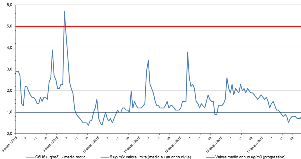
Benzene - C 6 H 6 Stazione di rilevamento di Sambruson, periodo: 08 giu 2015 - 14 giu 2015
