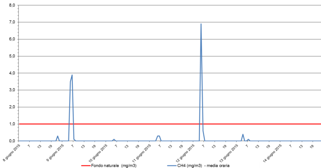
Metano - CH 4 Stazione di rilevamento di Sambruson, periodo: 08 giu 2015 - 14 giu 2015
