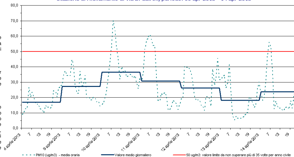
PM10 Stazione di rilevamento di via B. Cairoli, periodo: 08 apr 2013 - 14 apr 2013
