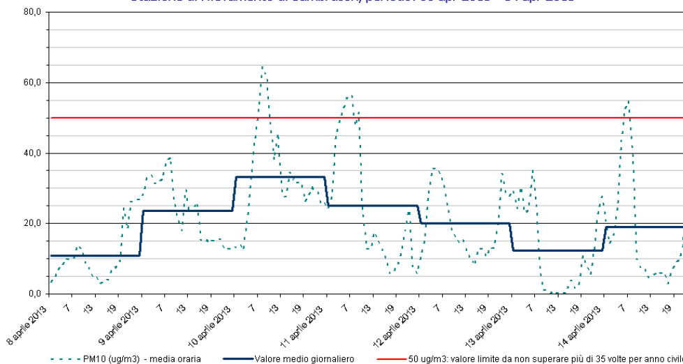
PM10 Stazione di rilevamento di Sambruson, periodo: 08 apr 2013 - 14 apr 2013
