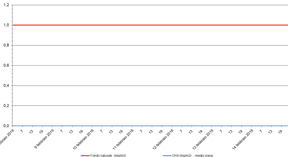
Metano - CH 4 Stazione di rilevamento di via B. Cairolì, periodo: 08 feb 2016 - 14 feb 2016
