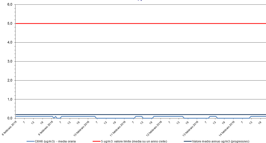
Benzene - C 6 H 6 Stazione di rilevamento di Sambruson, periodo: 08 feb 2016 - 14 feb 2016
