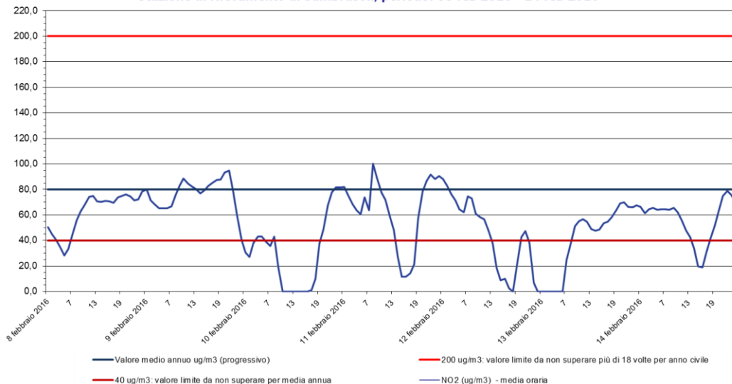
Biossido di azoto - NO 2 Stazione di rilevamento di Sambruson, periodo: 08 feb 2016 - 14 feb 2016
