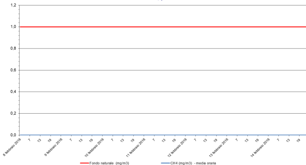
Metano - CH 4 Stazione di rilevamento di Sambruson, periodo: 08 feb 2016 - 14 feb 2016
