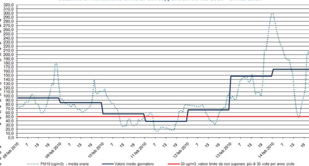
PM10 Stazione di rilevamento di via B. Cairoli, periodo: 08 feb 2010 - 14 feb 2010
