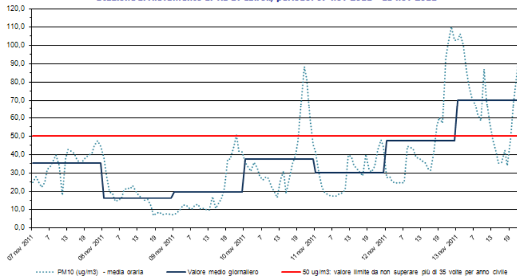
PM10 Stazione di rilevamento di via B. Cairoli, periodo: 07 nov 2011 - 13 nov 2011
