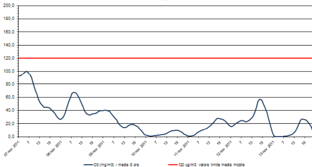
Ozono - O 3 Stazione di rilevamento di via B. Cairoli, periodo: 07 nov 2011 - 13 nov 2011
