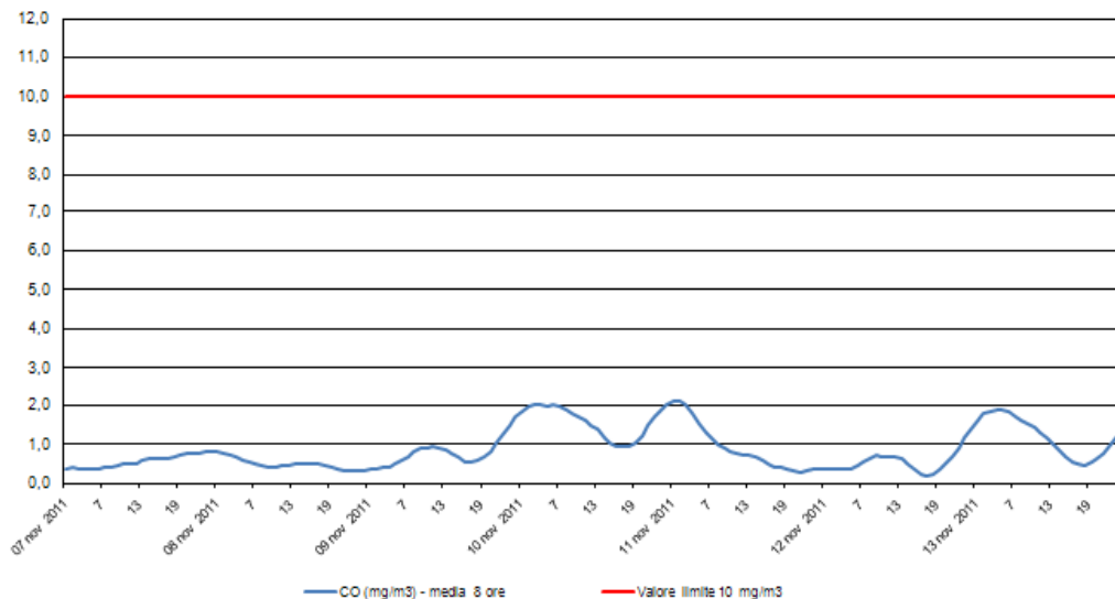
Monossido di Carbonio - CO Stazione di rilevamento di via B. Cairoli, periodo: 07 nov 2011 - 13 nov 2011
