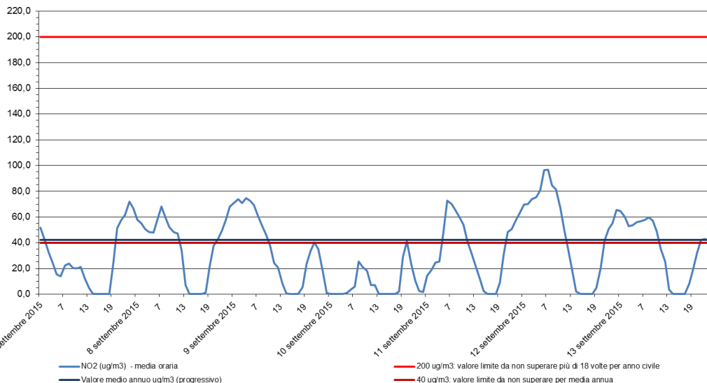
Biossido di azoto - NO 2 Stazione di rilevamento di via B. Cairoli, periodo: 07 set 2015 - 13 set 2015
