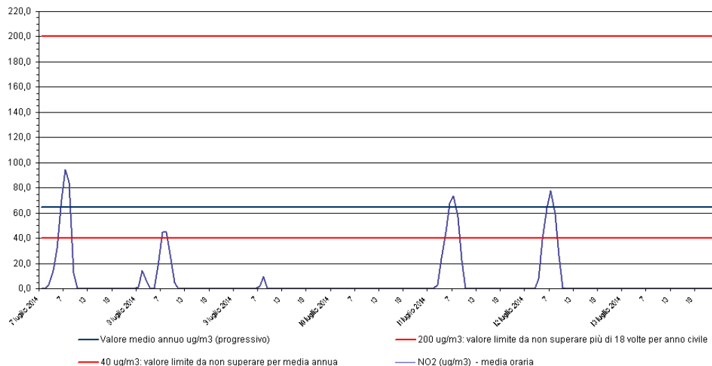
Biossido di azoto - NO 2 Stazione di rilevamento di Sambruson, periodo: 07 lug 2014 - 13 lug 2014
