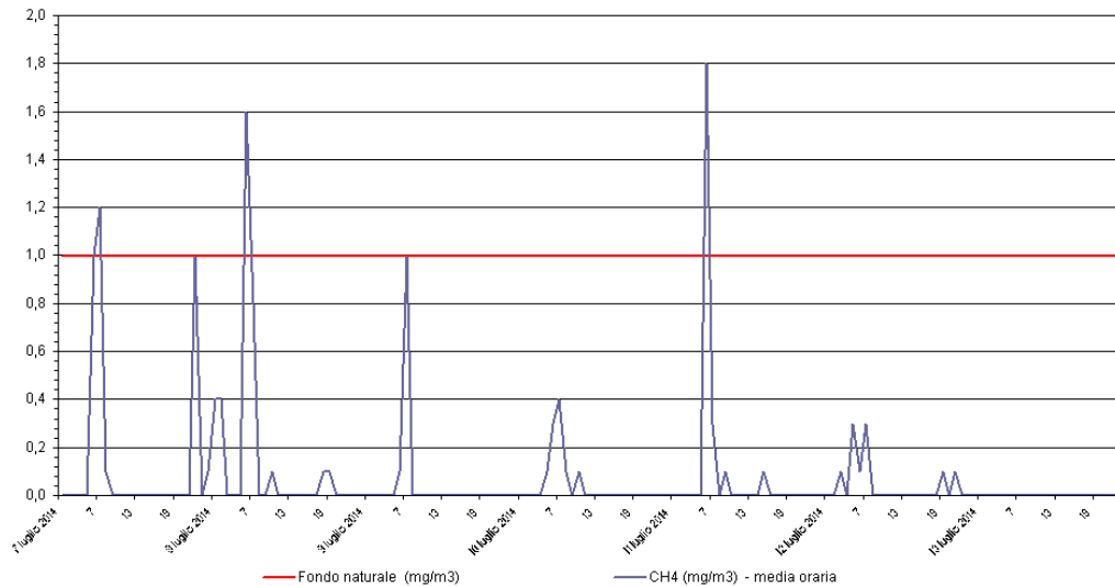
Metano - CH 4 Stazione di rilevamento di Sambruson, periodo: 07 lug 2014 - 13 lug 2014
