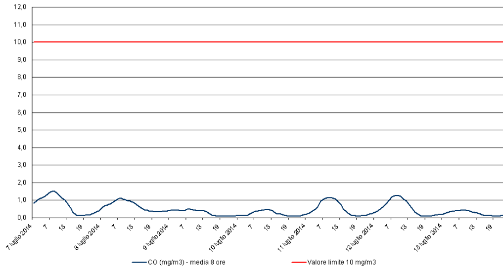
Monossido di Carbonio - CO Stazione di rilevamento di Sambruson, periodo: 07 lug 2014 - 13 lug 2014
