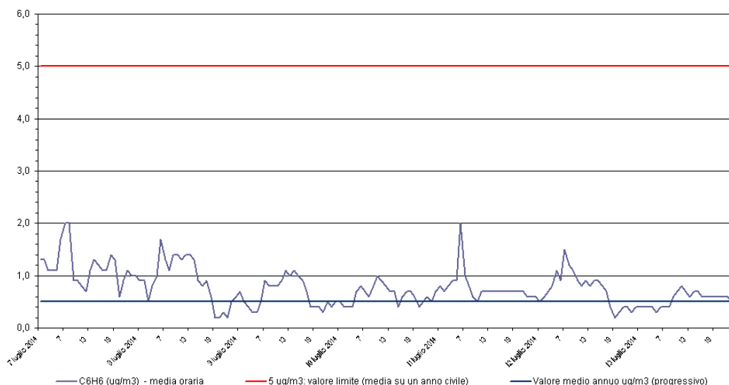
Benzene - C 6 H 6 Stazione di rilevamento di Sambruson, periodo: 07 lug 2014 - 13 lug 2014
