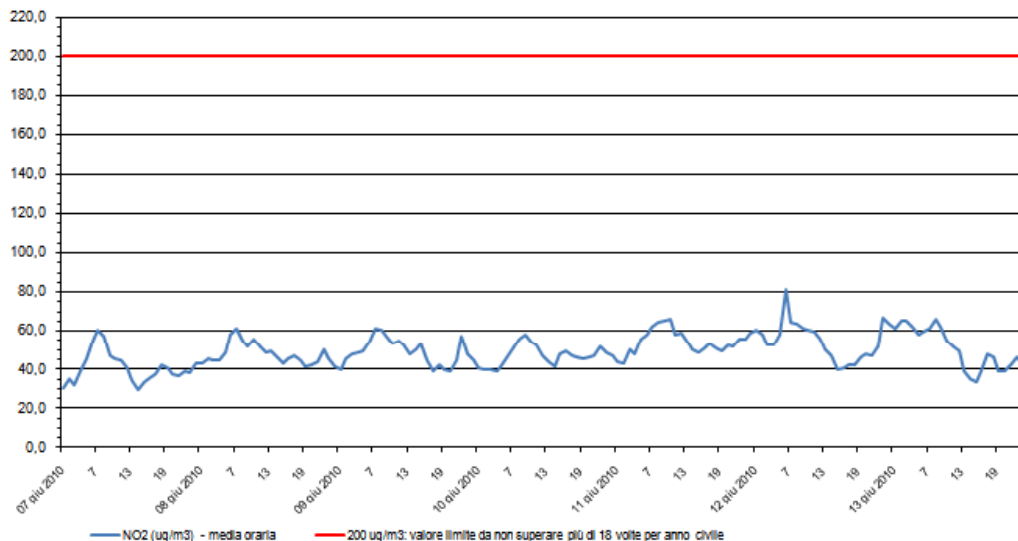
Biossido di azoto - NO 2 Stazione di rilevamento di via B. Cairoli, periodo 07 giu 2010 - 13 giu 2010
