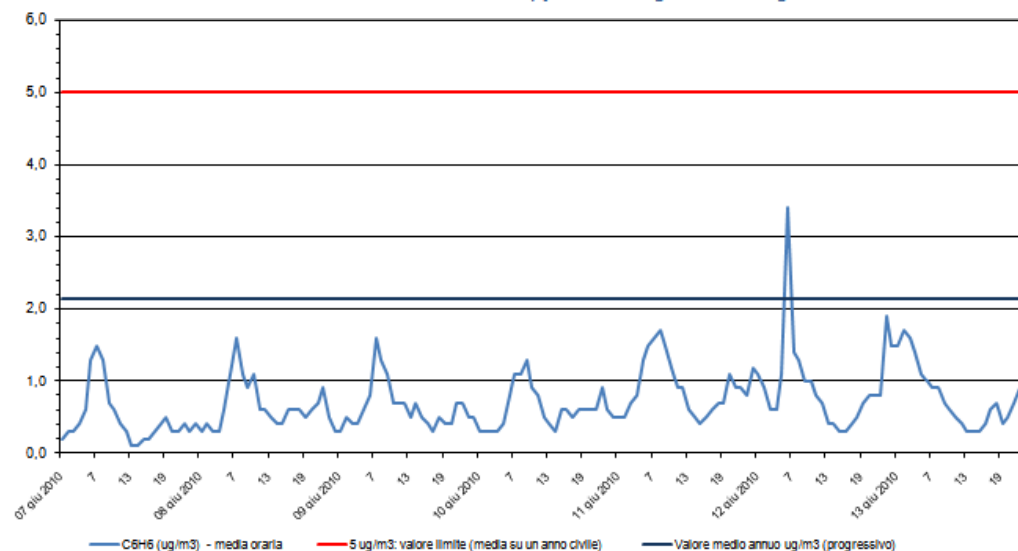
Benzene - C 6 H 6 Stazione di rilevamento di via B. Cairoli, periodo: 07 giu 2010 - 13 giu 2010
