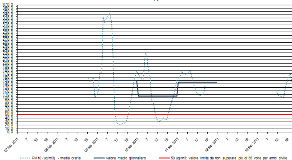
PM10 Stazione di rilevamento di via B. Cairoli, periodo: 07 feb 2011 - 13 feb 2011
