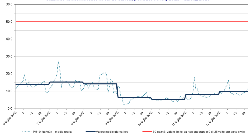
PM10 Stazione di rilevamento di via B. Cairoli, periodo: 06 lug 2015 - 12 lug 2015
