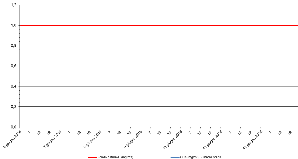
Metano - CH 4 Stazione di rilevamento di via B. Cairoli, periodo: 06 giu 2016 - 12 giu 2016
