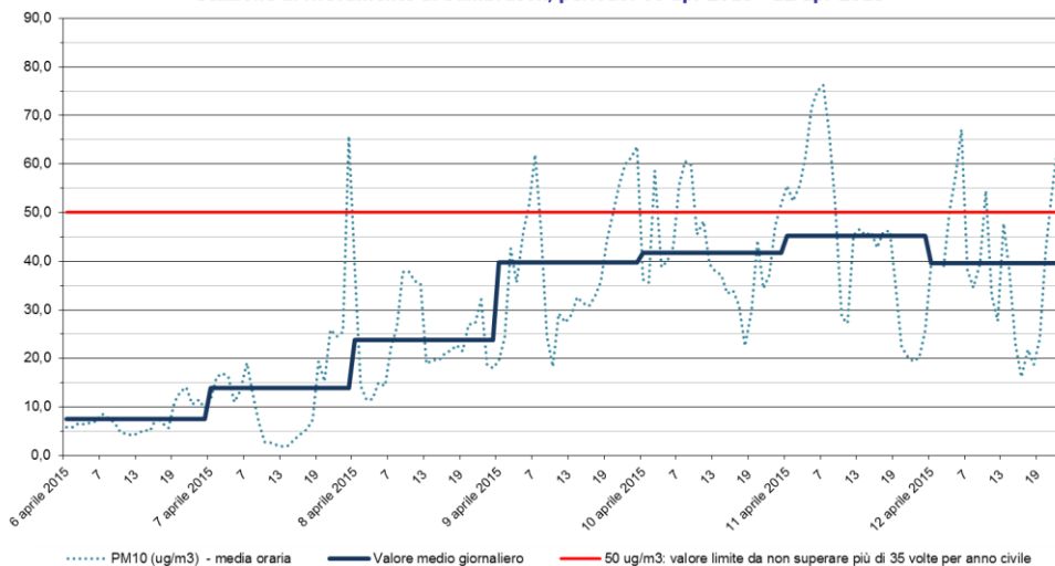
PM10 Stazione di rilevamento di Sambruson, periodo: 06 apr 2015 - 12 apr 2015
