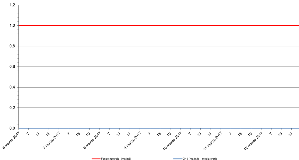
Metano - CH 4 Stazione di rilevamento di via B. Cairoli, periodo: 06 mar 2017 - 12 mar 2017
