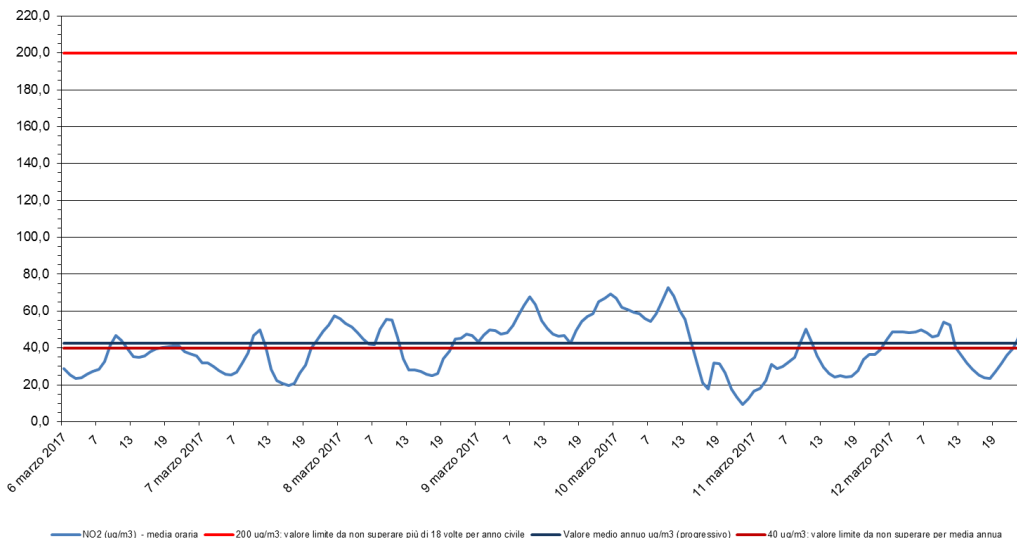
Biossido di azoto - NO 2 Stazione di rilevamento di via B. Cairoli, periodo: 06 mar 2017 - 12 mar 2017
