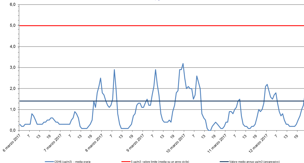
Benzene - C 6 H 6 Stazione di rilevamento di via B. Cairoli, periodo: 06 mar 2017 - 12 mar 2017
