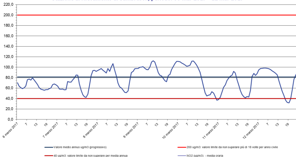
Biossido di azoto - NO 2 Stazione di rilevamento di Sambruson, periodo: 06 mar 2017 - 12 mar 2017
