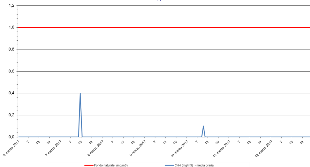
Metano - CH 4 Stazione di rilevamento di Sambruson, periodo: 06 mar 2017 - 12 mar 2017
