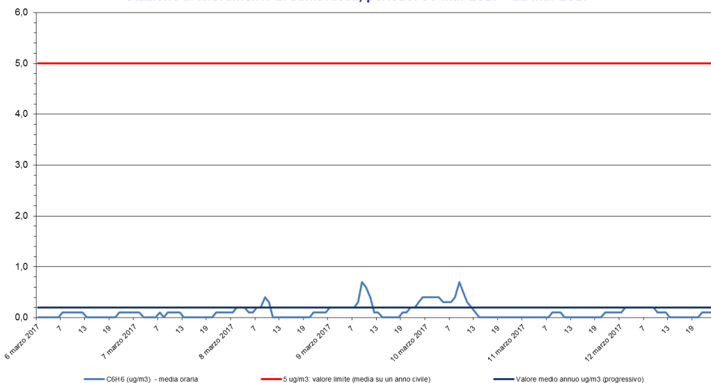
Benzene - C 6 H 6 Stazione di rilevamento di Sambruson, periodo: 06 mar 2017 - 12 mar 2017
