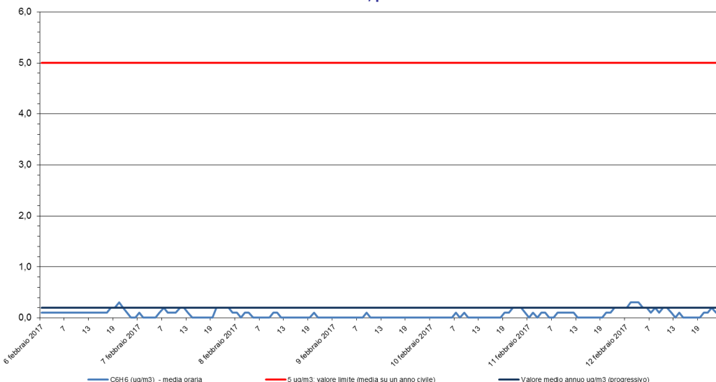
Benzene - C 6 H 6 Stazione di rilevamento di Sambruson, periodo: 06 feb 2017 - 12 feb 2017
