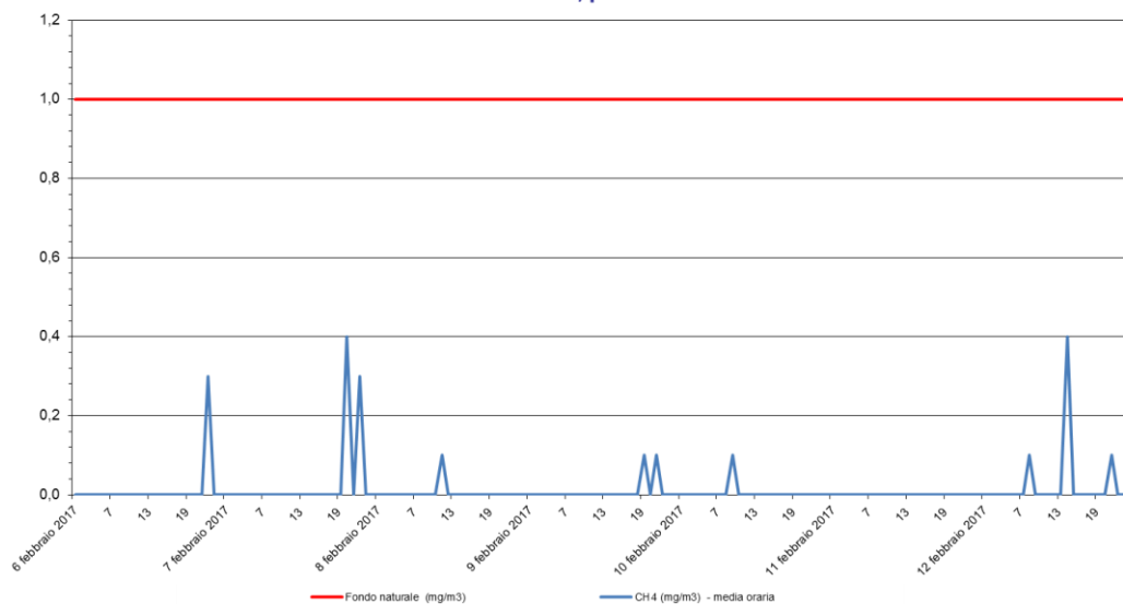
Metano - CH 4 Stazione di rilevamento di Sambruson, periodo: 06 feb 2017 - 12 feb 2017
