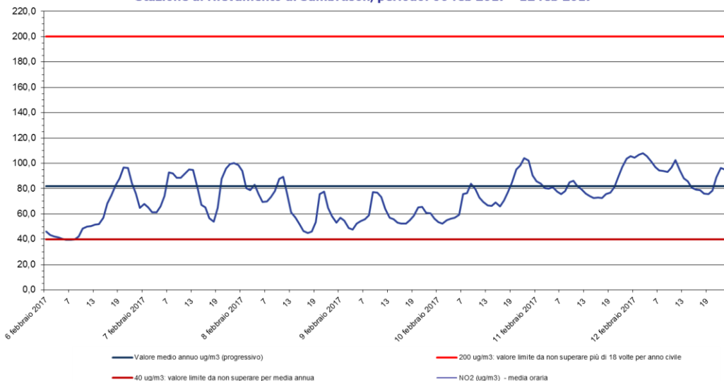
Biossido di azoto - NO 2 Stazione di rilevamento di Sambruson, periodo: 06 feb 2017 - 12 feb 2017
