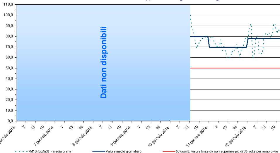
PM10 Stazione di rilevamento di via B. Cairoli, periodo: 06 gen 2014 - 12 gen 2014
