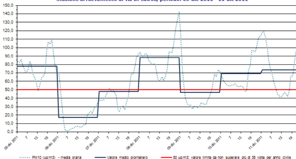
PM10 Stazione di rilevamento di via B. Cairoli, periodo: 05 dic 2011 - 11 dic 2011
