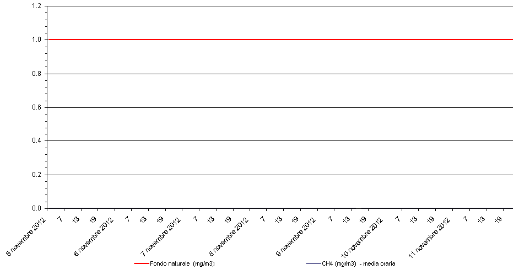
Metano - CH 4 Stazione di rilevamento di via B. Cairoli, periodo: 05 nov 2012 - 11 nov 2012
