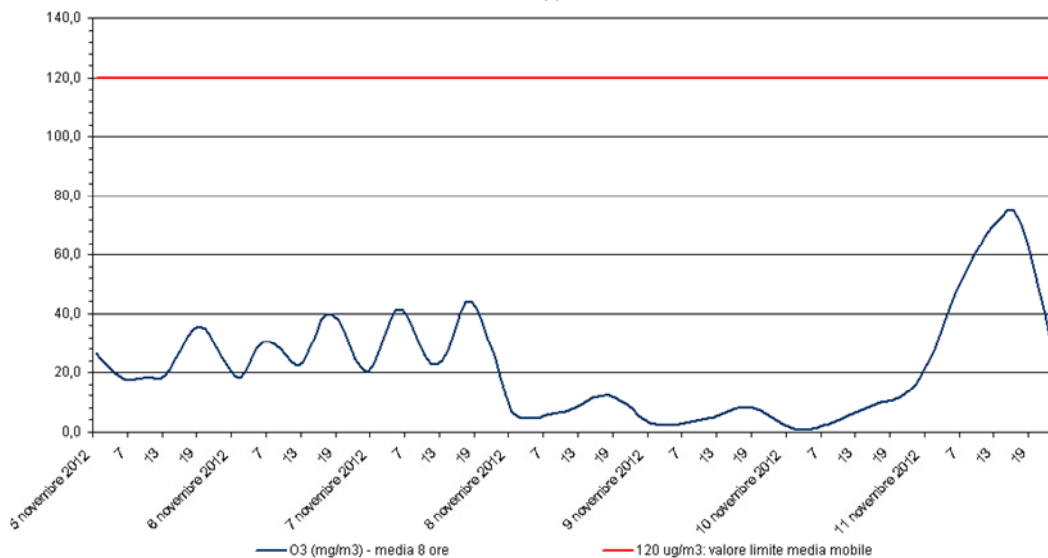
Ozono - O 3 Stazione di rilevamento di Sambruson, periodo: 05 nov 2012 - 11 nov 2012
