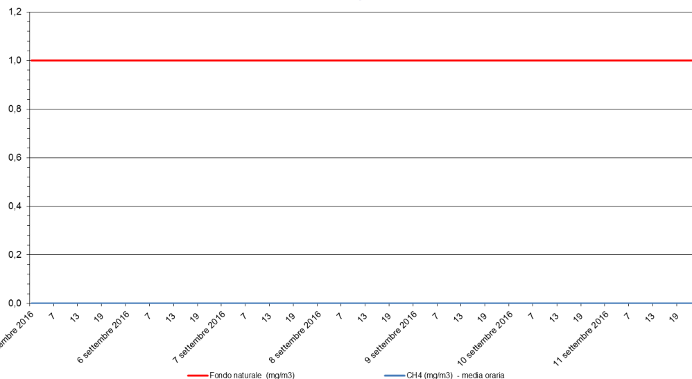
Metano - CH 4 Stazione di rilevamento di via B. Cairoli, periodo: 05 set 2016 - 11 set 2016
