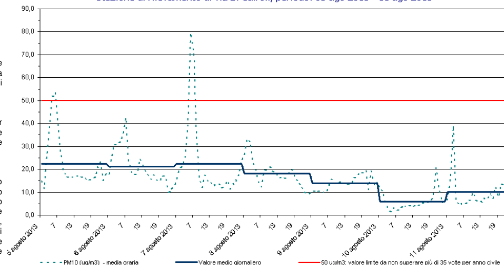
PM10 Stazione di rilevamento di via B. Cairoli, periodo: 05 ago 2013 - 11 ago 2013
