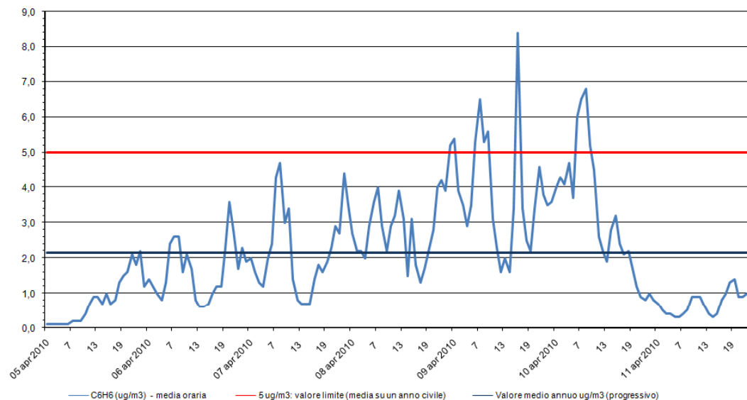
Benzene - C 6 H 6 Stazione di rilevamento di via B. Cairoli, periodo: 05 apr 2010 al 11 apr 2010
