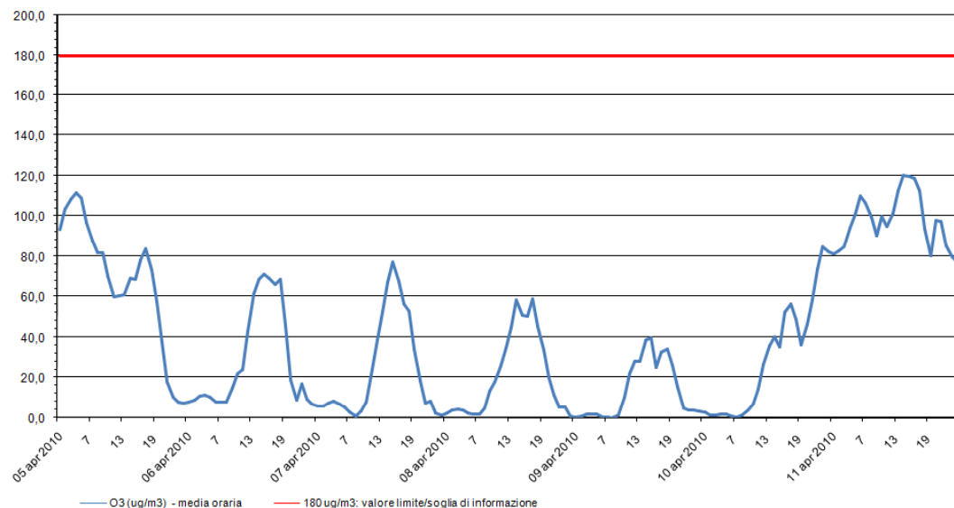
Ozono - O3 Stazione di rilevamento di via B. Cairoli, periodo: 05 apr 2010 al 11 apr 2010
