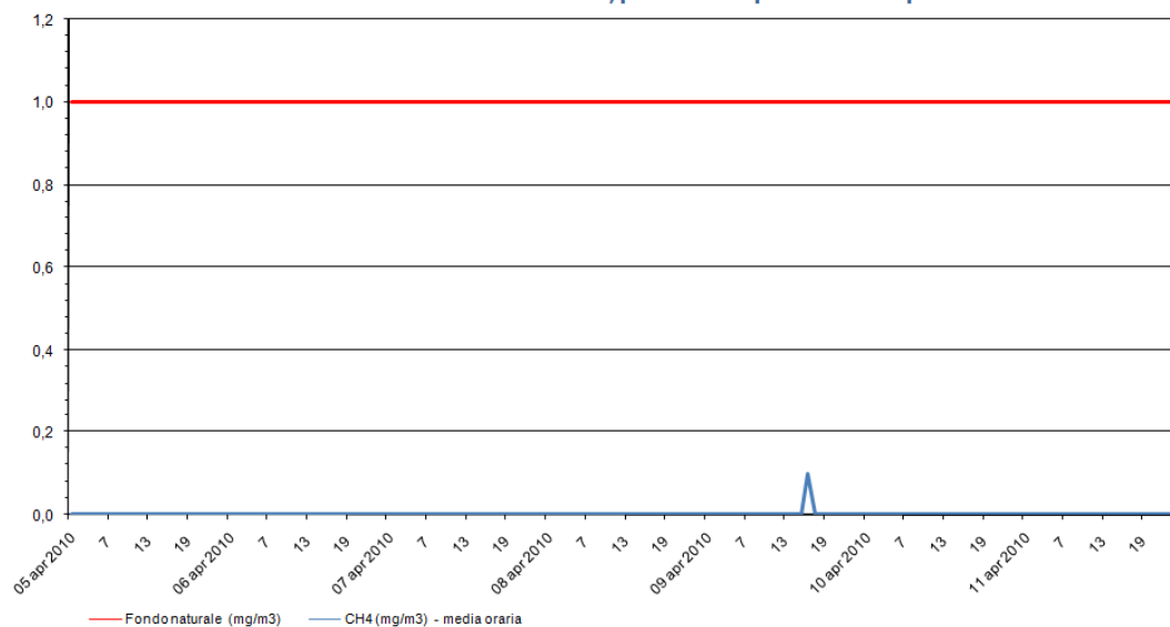
Metano - CH 4 Stazione di rilevamento di via B. Cairoli, periodo: 05 apr 2010 al 11 apr 2010
