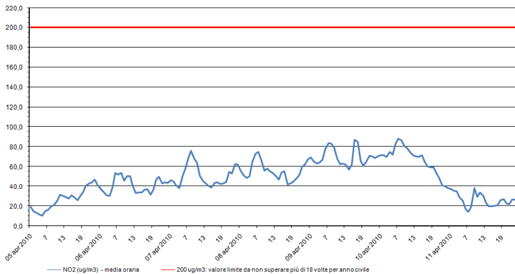
Biossido di azoto - NO 2 Stazione di rilevamento di via B. Cairoli, periodo: 05 apr 2010 al 11 apr 2010
