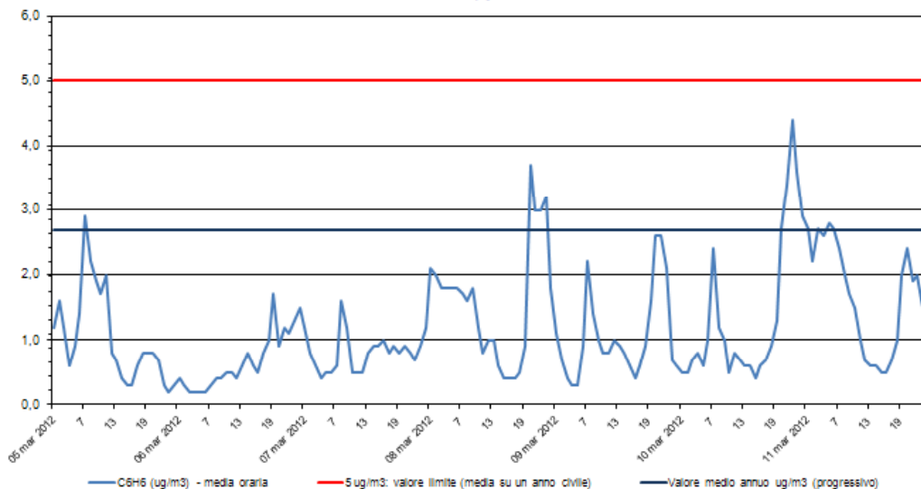
Benzene - C 6 H 6 Stazione di rilevamento di via B. Cairoli, periodo: 05 mar 2012- 11 mar 2012
