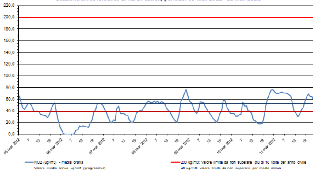
Biossido di azoto - NO 2 Stazione di rilevamento di via B. Cairoli, periodo: 05 mar 2012- 11 mar 2012
