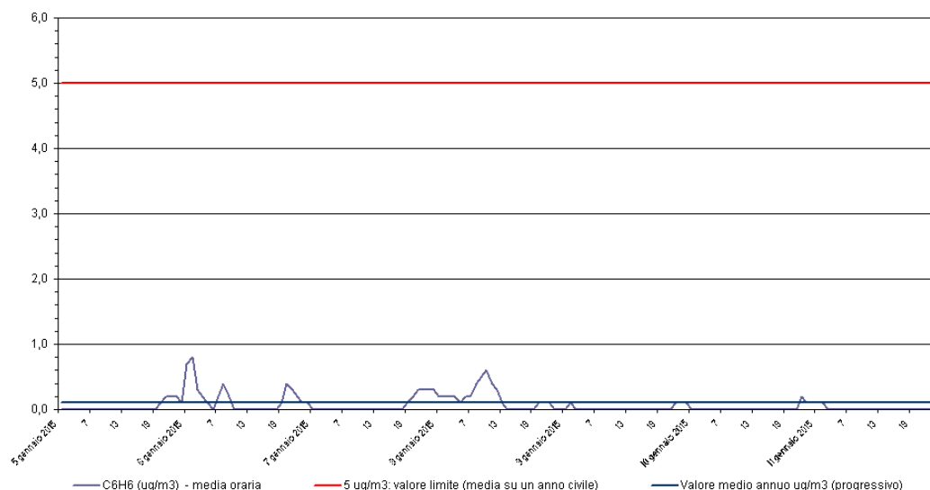
Benzene - C 6 H 6 Stazione di rilevamento di Sambruson, periodo: 05 gen 2015 - 11 gen 2015
