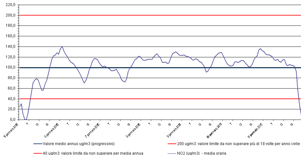
Biossido di azoto - NO 2 Stazione di rilevamento di Sambruson, periodo: 05 gen 2015 - 11 gen 2015
