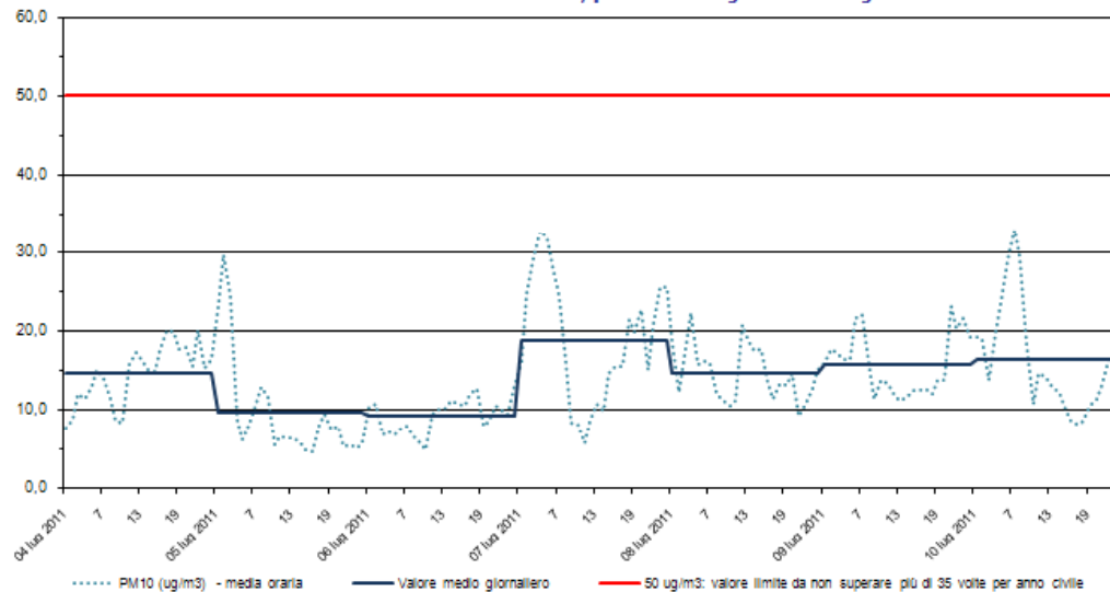
PM10 Stazione di rilevamento di via B. Cairoli, periodo: 04 lug 2011 - 10 lug 2011
