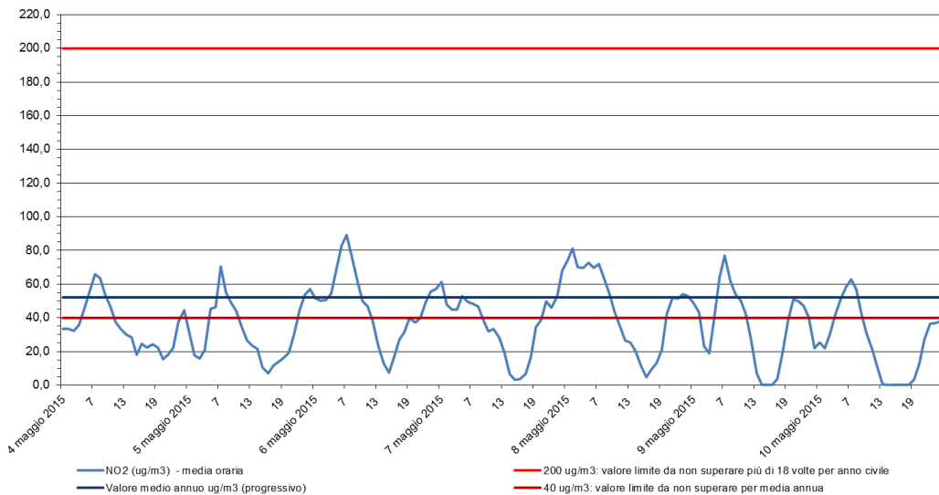
Biossido di azoto - NO 2 Stazione di rilevamento di via B. Cairoli, periodo: 04 mag 2015 - 10 mag 2015
