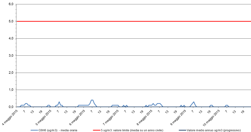
Benzene - C 6 H 6 Stazione di rilevamento di via B. Cairoli, periodo: 04 mag 2015 - 10 mag 2015
