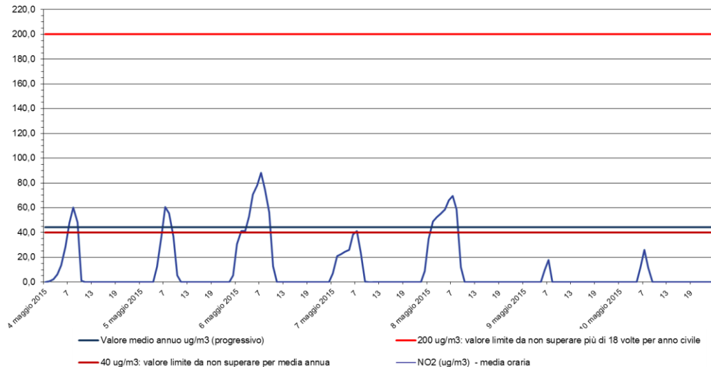
Biossido di azoto - NO2 Stazione di rilevamento di Sambruson, periodo: 04 mag 2015 - 10 mag 2015
