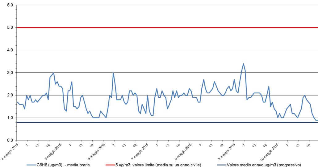
Benzene - C6H6 Stazione di rilevamento di Sambruson, periodo: 04 mag 2015 - 10 mag 2015
