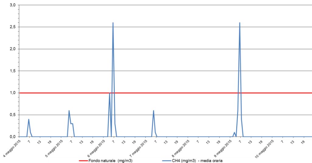
Metano - CH 4 Stazione di rilevamento di Sambruson, periodo: 04 mag 2015 - 10 mag 2015
