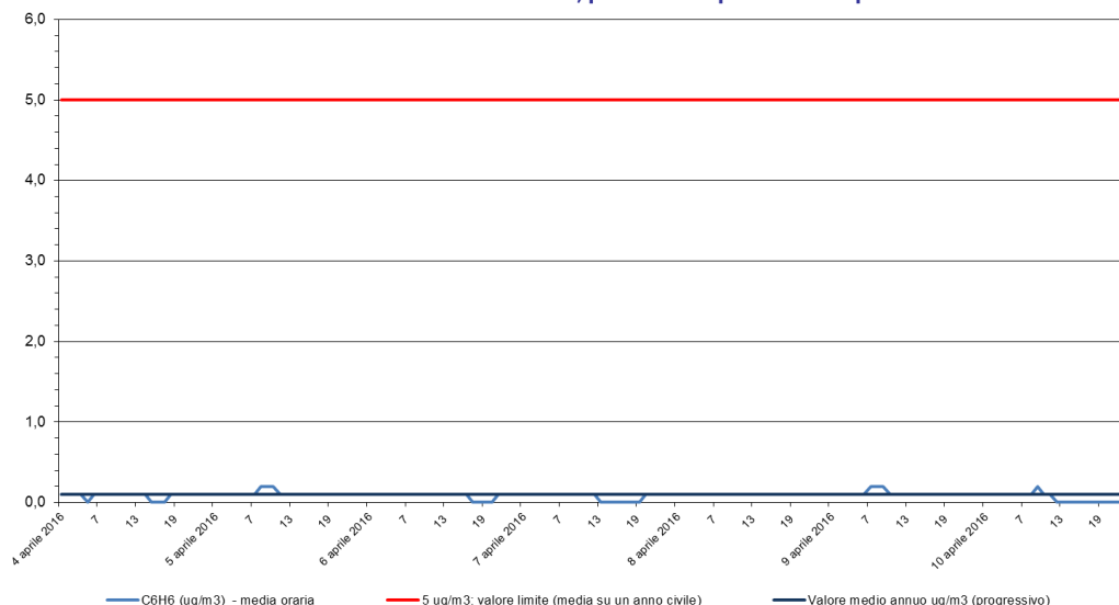
Benzene - C 6 H 6 Stazione di rilevamento di Sambruson, periodo: 04 apr 2016 - 10 apr 2016
