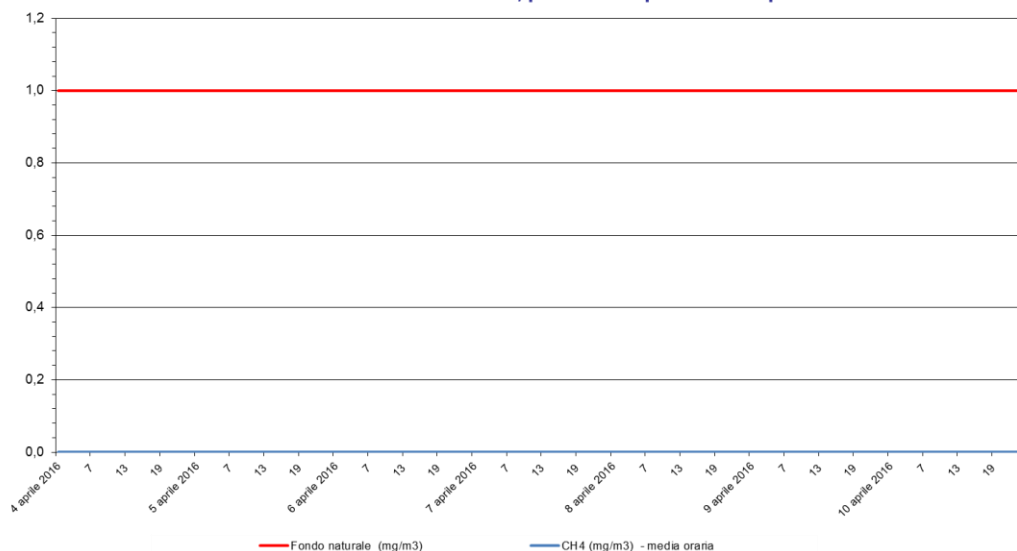
Metano - CH 4 Stazione di rilevamento di Sambruson, periodo: 04 apr 2016 - 10 apr 2016
