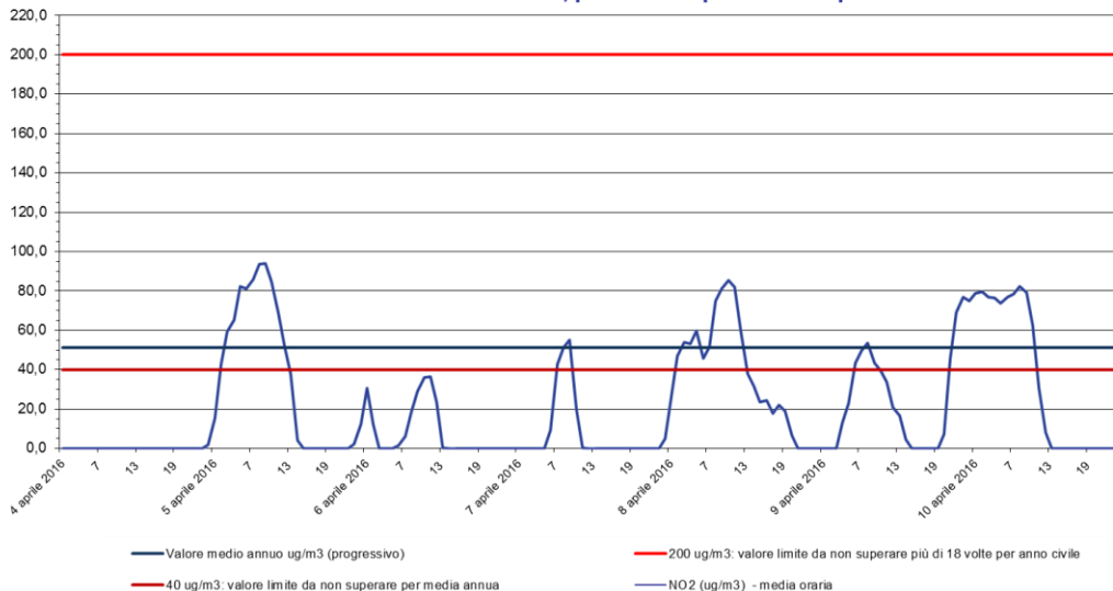
Biossido di azoto - NO 2 Stazione di rilevamento di Sambruson, periodo: 04 apr 2016 - 10 apr 2016
