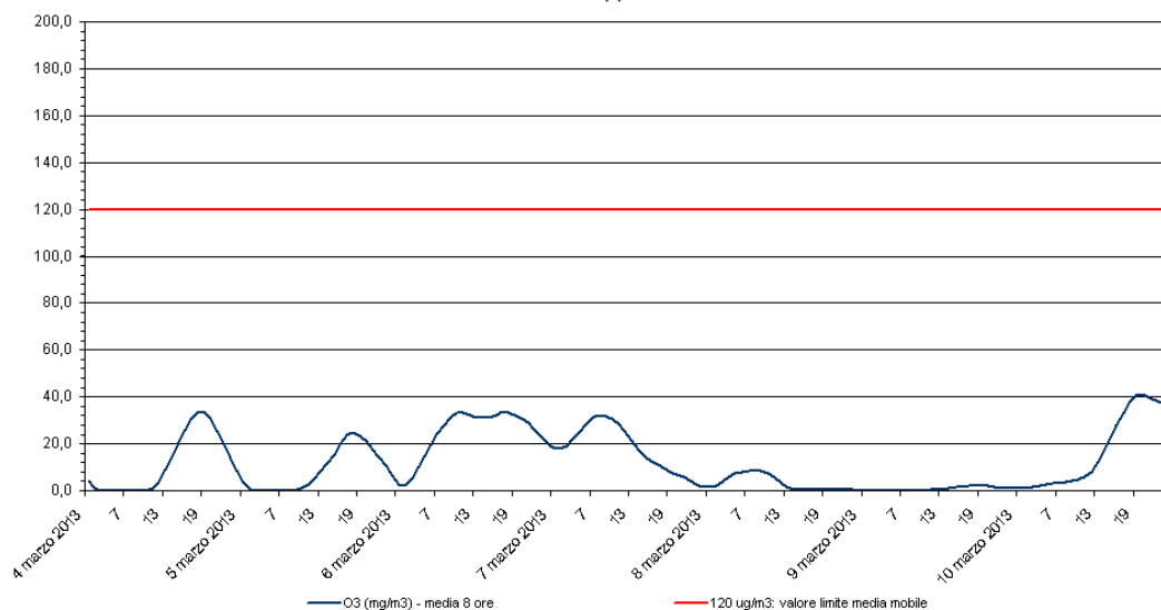
Ozono - O 3 Stazione di rilevamento di via B. Cairoli, periodo: 04 mar 2013 - 10 mar 2013
