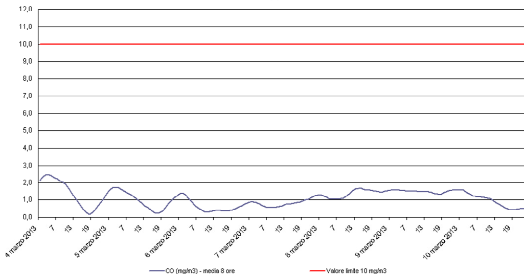
Monossido di Carbonio - CO Stazione di rilevamento di via B. Cairoli, periodo: 04 mar 2013 - 10 mar 2013
