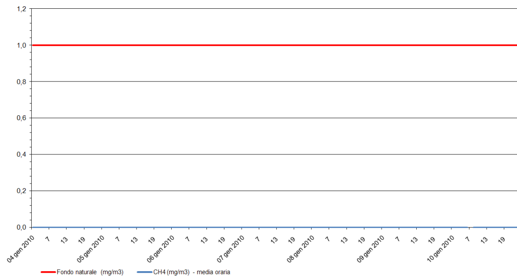
Metano - CH 4 Stazione di rilevamento di via F.lli Bandiera, periodo: 04 gen 2010 - 10 gen 2010
