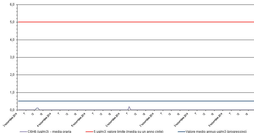
Benzene - C 6 H 6 Stazione di rilevamento di Sambruson, periodo: 03 nov 2014 - 09 nov 2014
