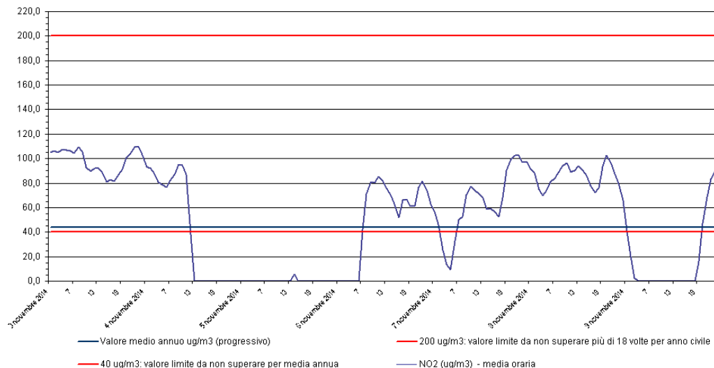
Biossido di azoto - NO 2 Stazione di rilevamento di Sambruson, periodo: 03 nov 2014 - 09 nov 2014
