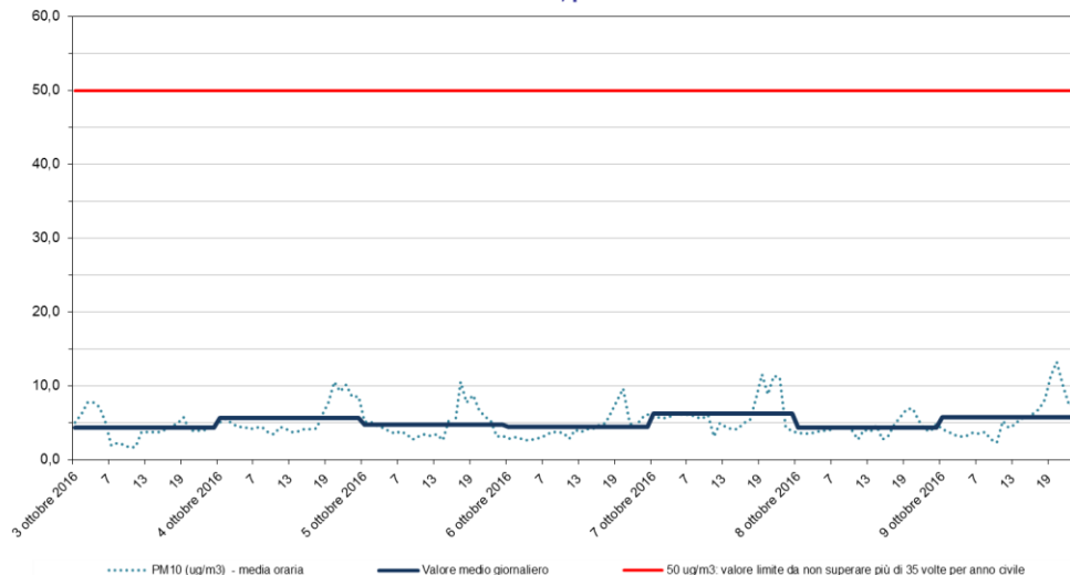
PM10 Stazione di rilevamento di via B. Cairoli, periodo: 03 ott 2016 - 09 ott 2016
